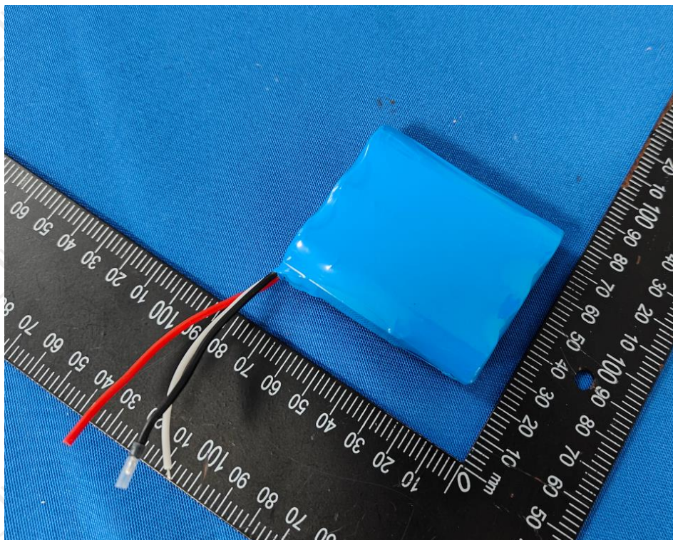
Picture 4. Back view of cell 图片 4. 电芯后视图
