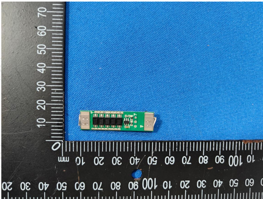
Picture 7. Front view of protection board 图片 7. 保护板前视图
