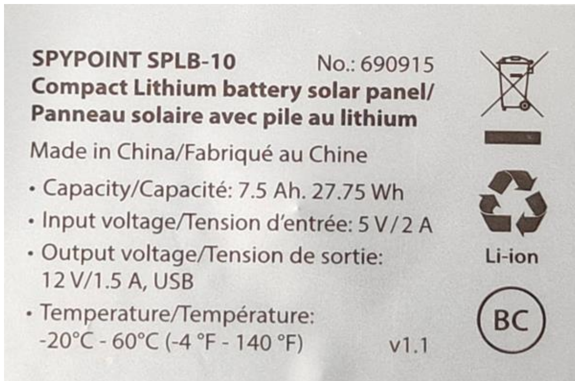
Picture 9. Label view 图片 9. 标签视图
